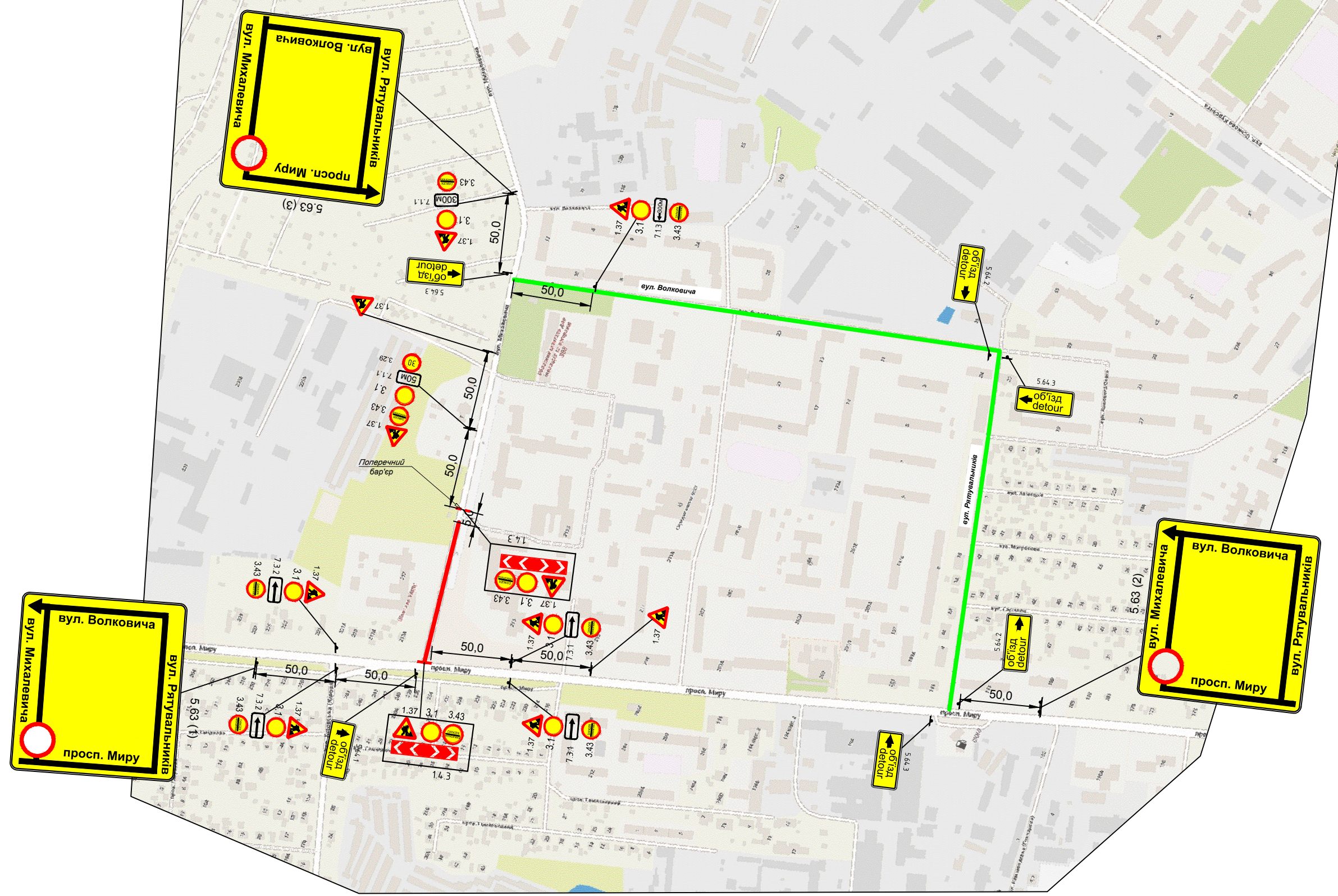
Схема організації дорожнього руху під час довгострокових стіціонарних дорожніх робіт у межах населеного пункту на період ремонту дорожнього покриття по вул. Михалевича на ділянці від просп. Миру 200м в напрямку вул. Курсанта Єськова в м. Чернігів
