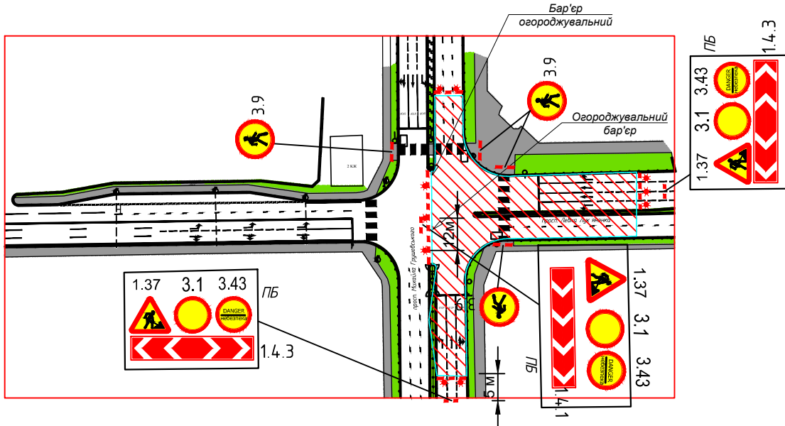
Схема організації дорожнього руху під час довгострокових стіціонарних дорожніх робіт у межах населеного пункту на період ремонту дорожнього покриття на перехресті просп. Левка Лук'яненка та просп. Грушевського (правий проїзд) в м. Чернігів
